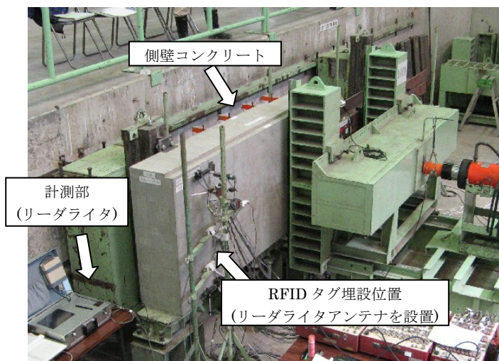
載荷試験によるセンサ RFID の確認試験状況
