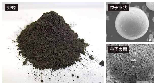
リチウムイオン電池の正極材料「ナノリチア」
