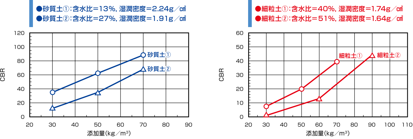
添加量とCBRの関係
