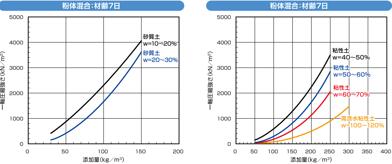
添加量と一軸圧縮強さの関係
