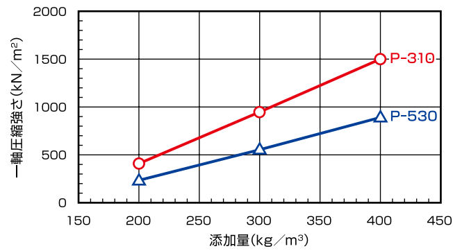
スラリー混合(W/C=70%):高有機質土
