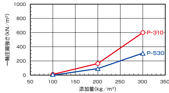
スラリー混合(W/C=60%):高有機質土
