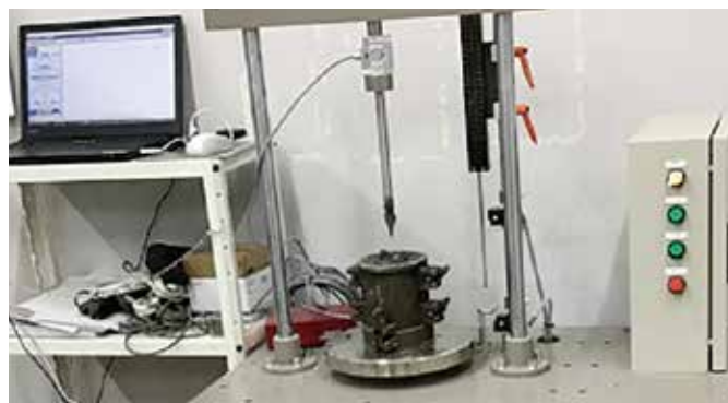
コーン貫入試験
