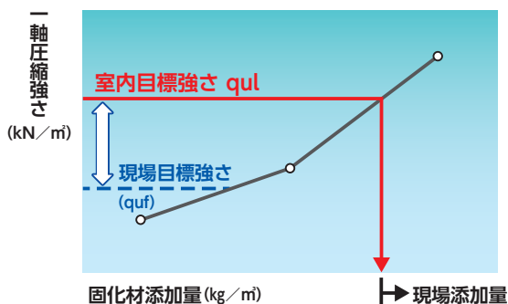
浅層改良の（現場/室内）強さ比
