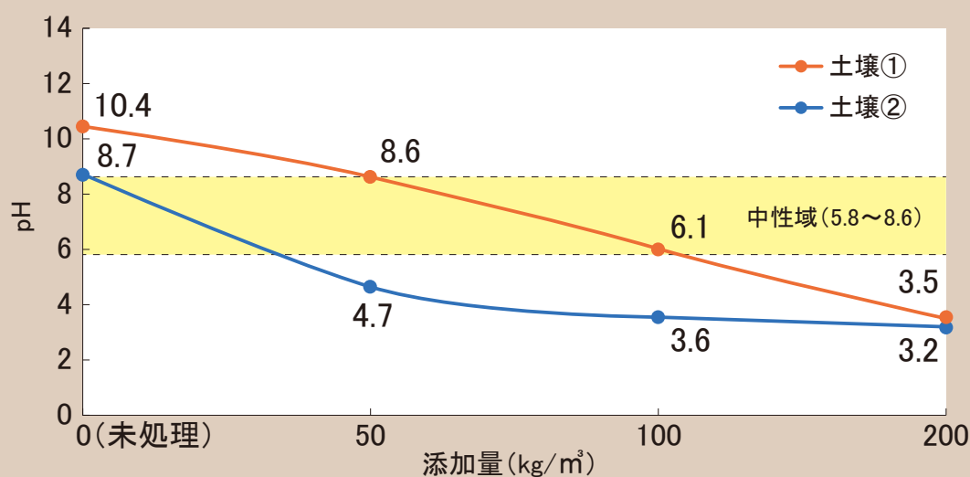
【硫酸第一鉄を土壌に添加した際のpH変化】
