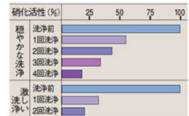
■ろ過材洗浄での硝化活性低下 (循環ろ過水槽・海水)
